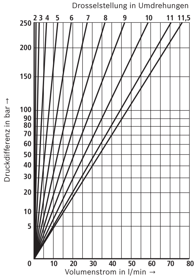
\Delta p - q_V -Kennlinien (Ausführung „1Q“)
